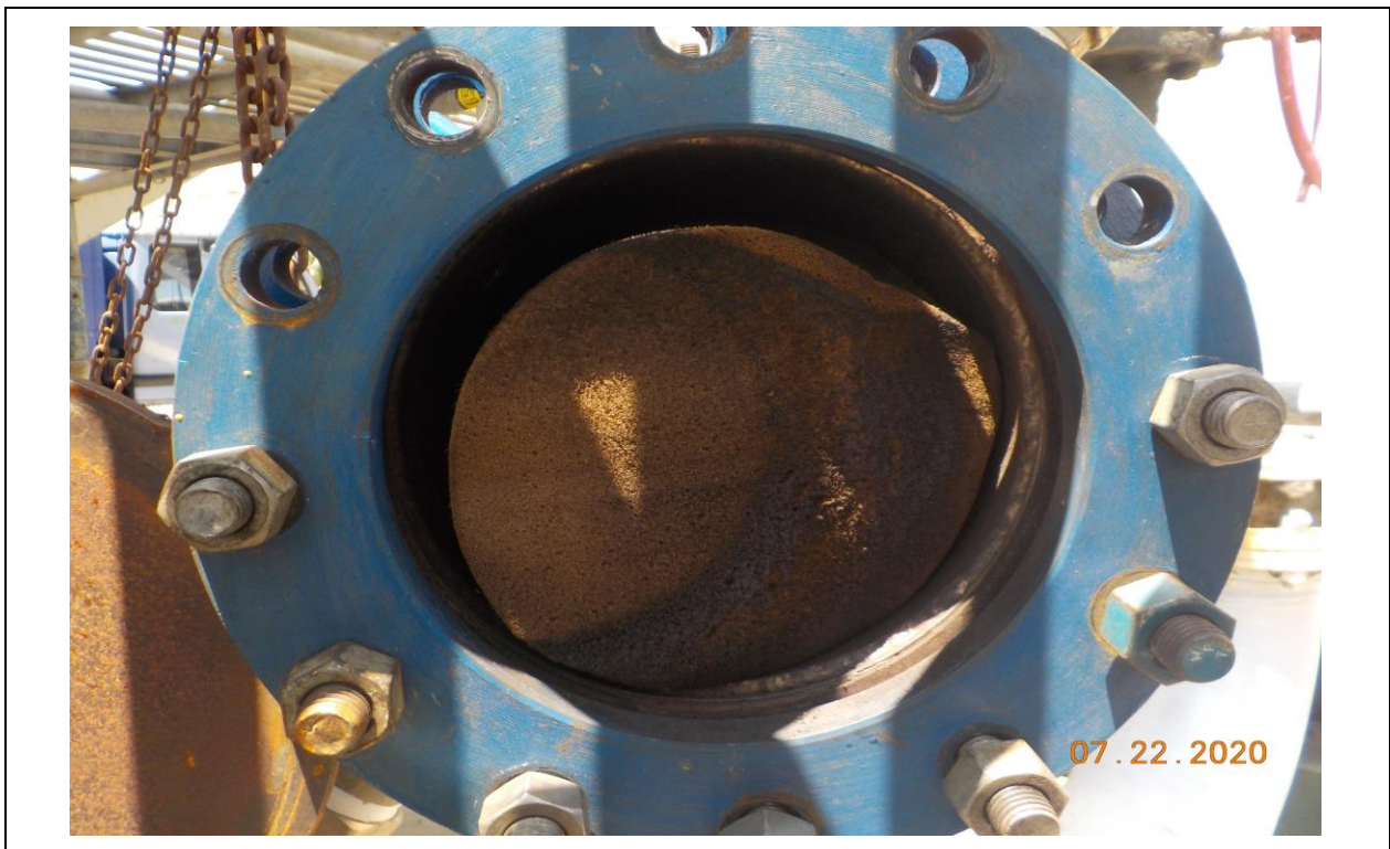
接收端接收 PIG 情況(5)
